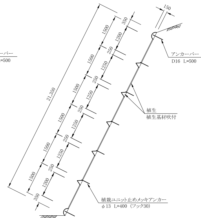
C-C 断面図 S = 1/100
