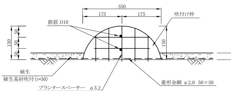
吹付け枠断面図 S = 1/10
