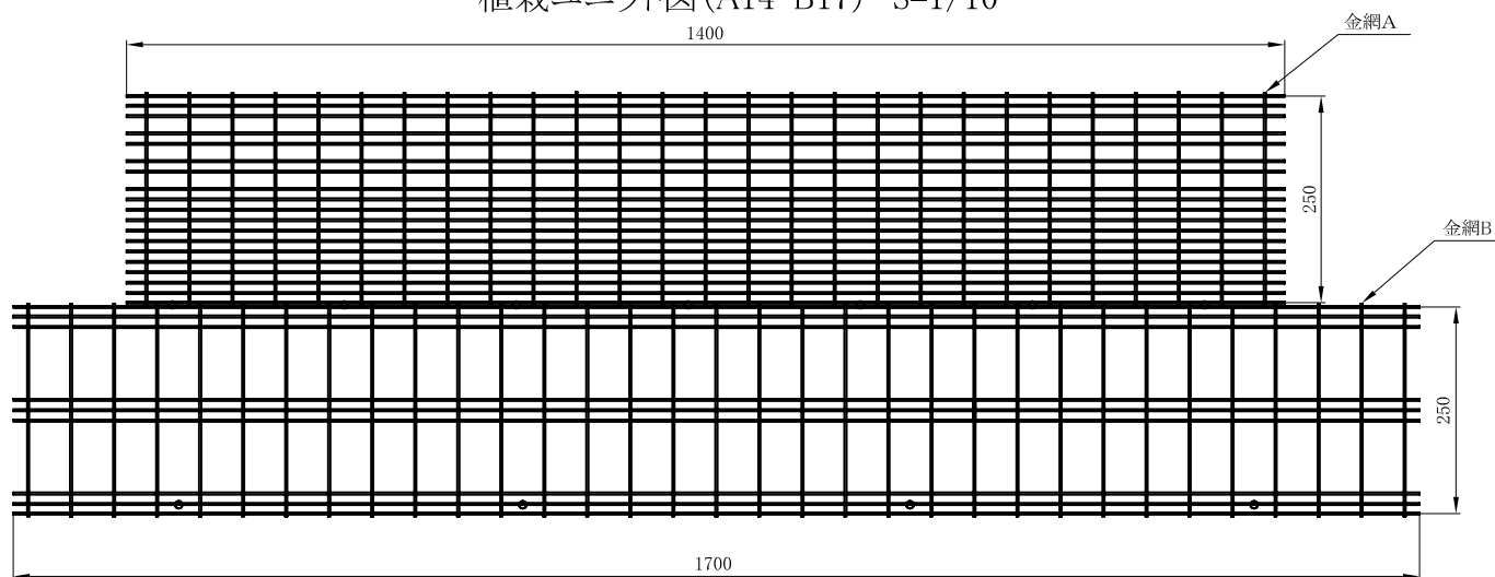
植栽ユニット図 (A14-B17) S=1/10
