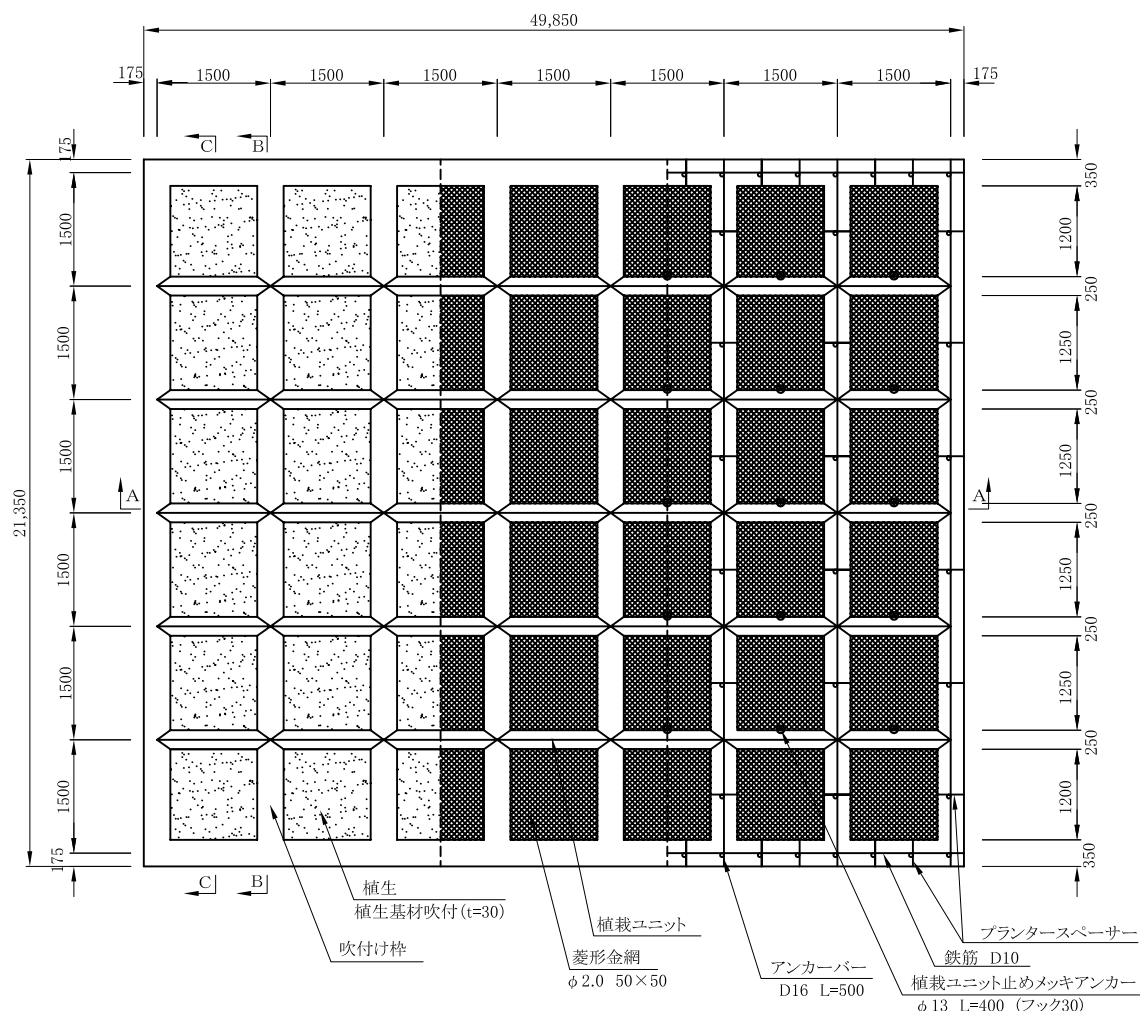
植栽ユニット図 (A14-B17) S=1/10
