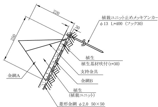
植栽ユニット断面図 S = 1/10
