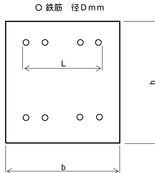
図-1 鉄筋の配置長 L
